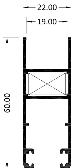
3752 HOJA PERIMETRAL H19 MM
