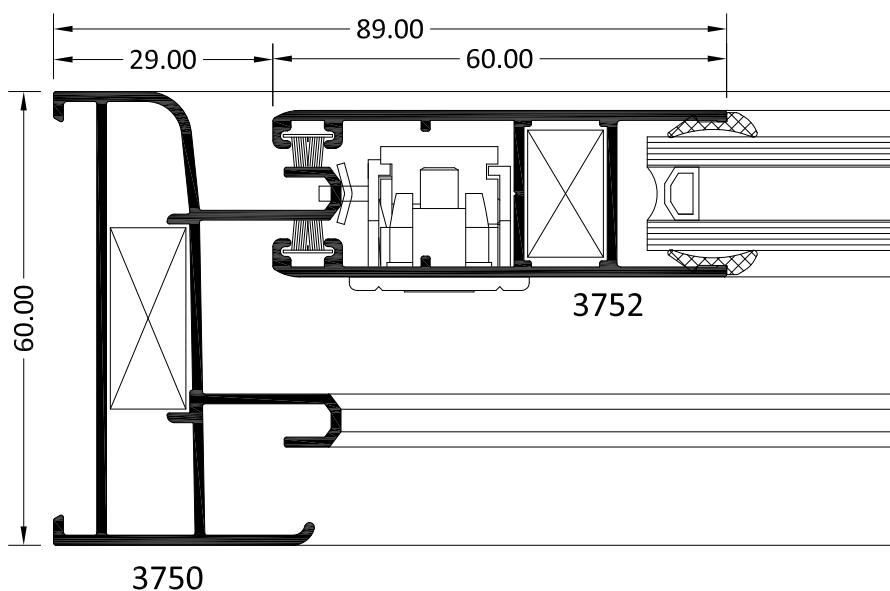
SECCIÓN S3
