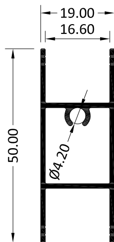
3758 TRAVESAÑO HUECO 16.6 MM
