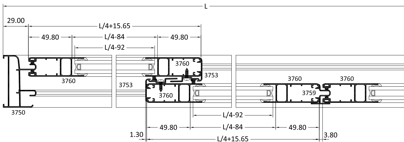
SECCIÓN HORIZONTAL A-A'
