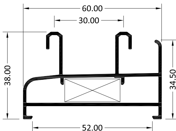
3750 CERCO PERIMETRAL
