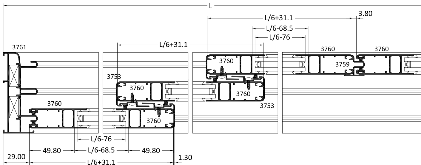
SECCIÓN HORIZONTAL A-A'
