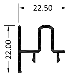
3759 CENTRO DE CUATRO HOJAS
