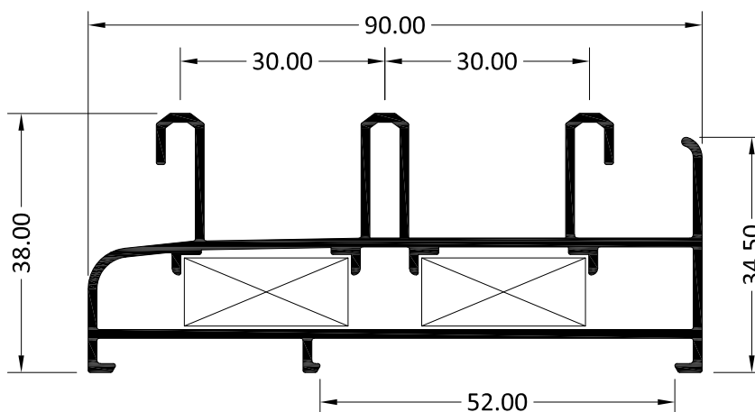
3761 CERCO PERIMETRAL TRES CARRILES
