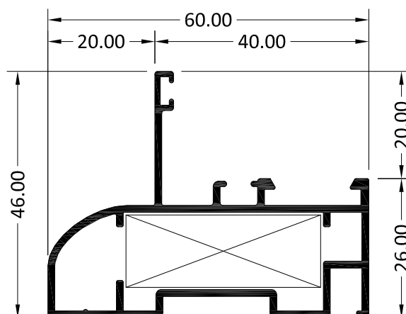
5662 FIJO MARCO 60 MM S-5600
