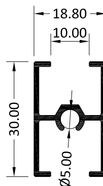
4122 TRAVESAÑO 30 HUECO 10 MM
