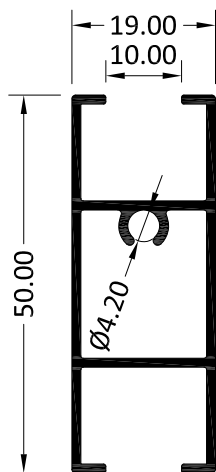
3757 TRAVESAÑO HUECO 10 MM
