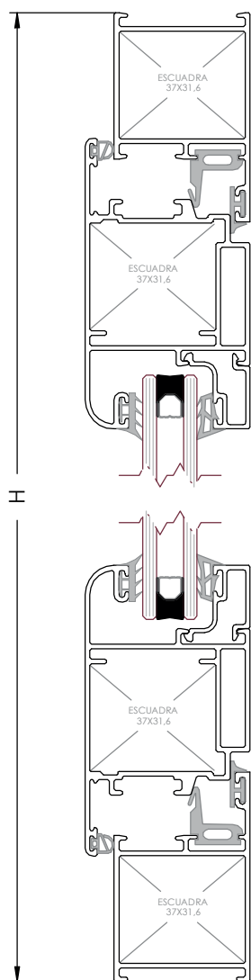
SECCIÓN VERTICAL 1:2
