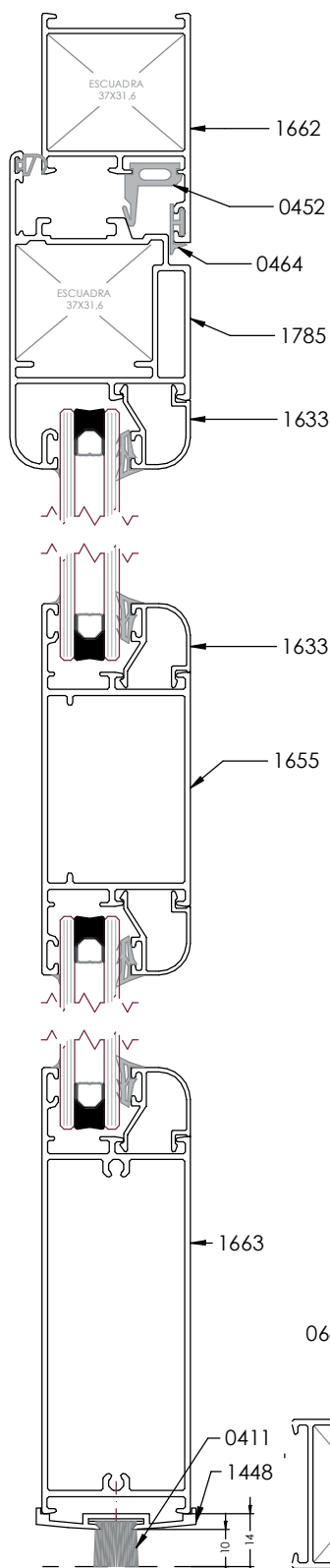
SECCIÓN VERTICAL 1:2
