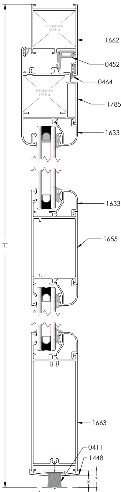
SECCIÓN VERTICAL 1:2
