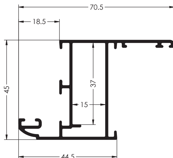
Ref. 1900(*) CERCO CURVO VENTANA CON SOLAPE
