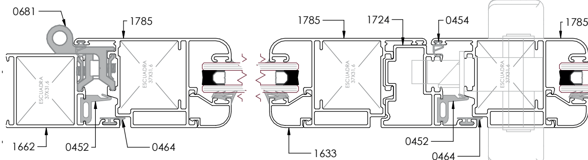
SECCIÓN HORIZONTAL 1:2
