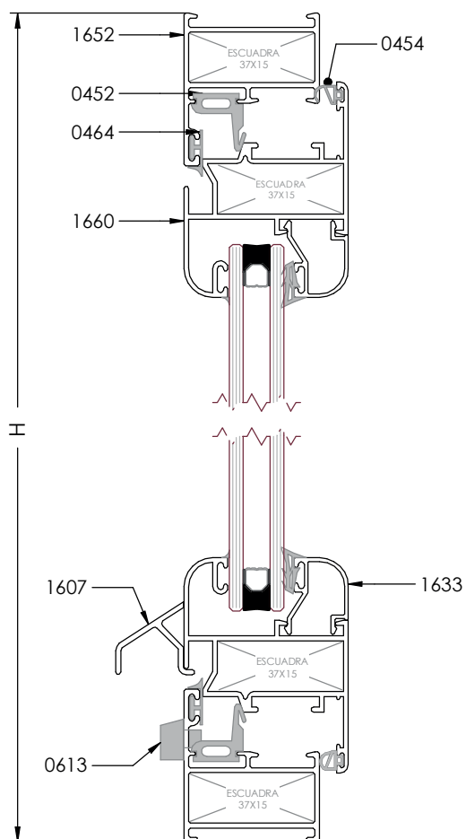
SECCIÓN VERTICAL 1:2
